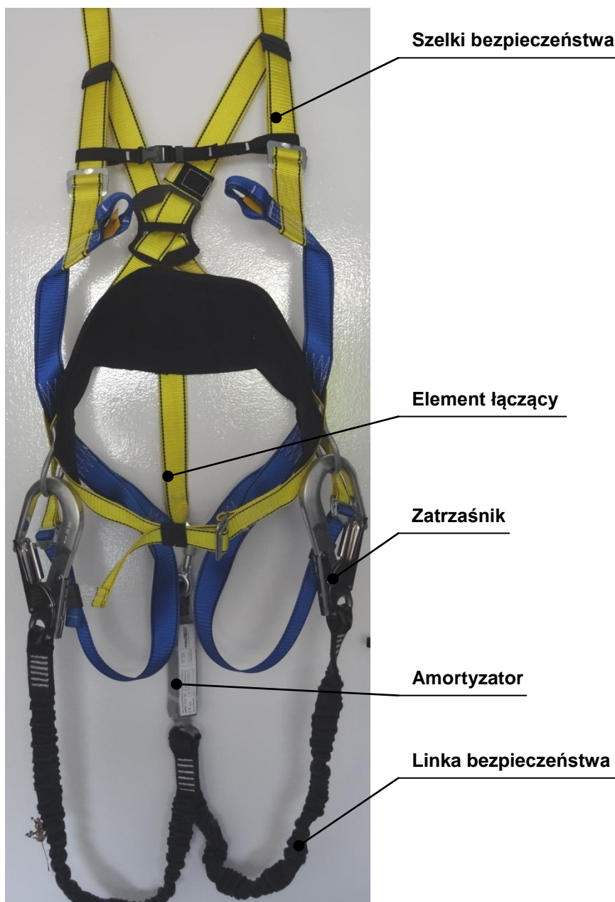
Rys. 1. Przykładowy zestaw zabezpieczający montera przed upadkiem z wysokości [1]
